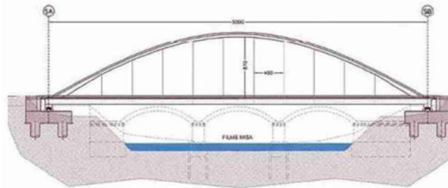
Il progetto del nuovo ponte del Coppetto
